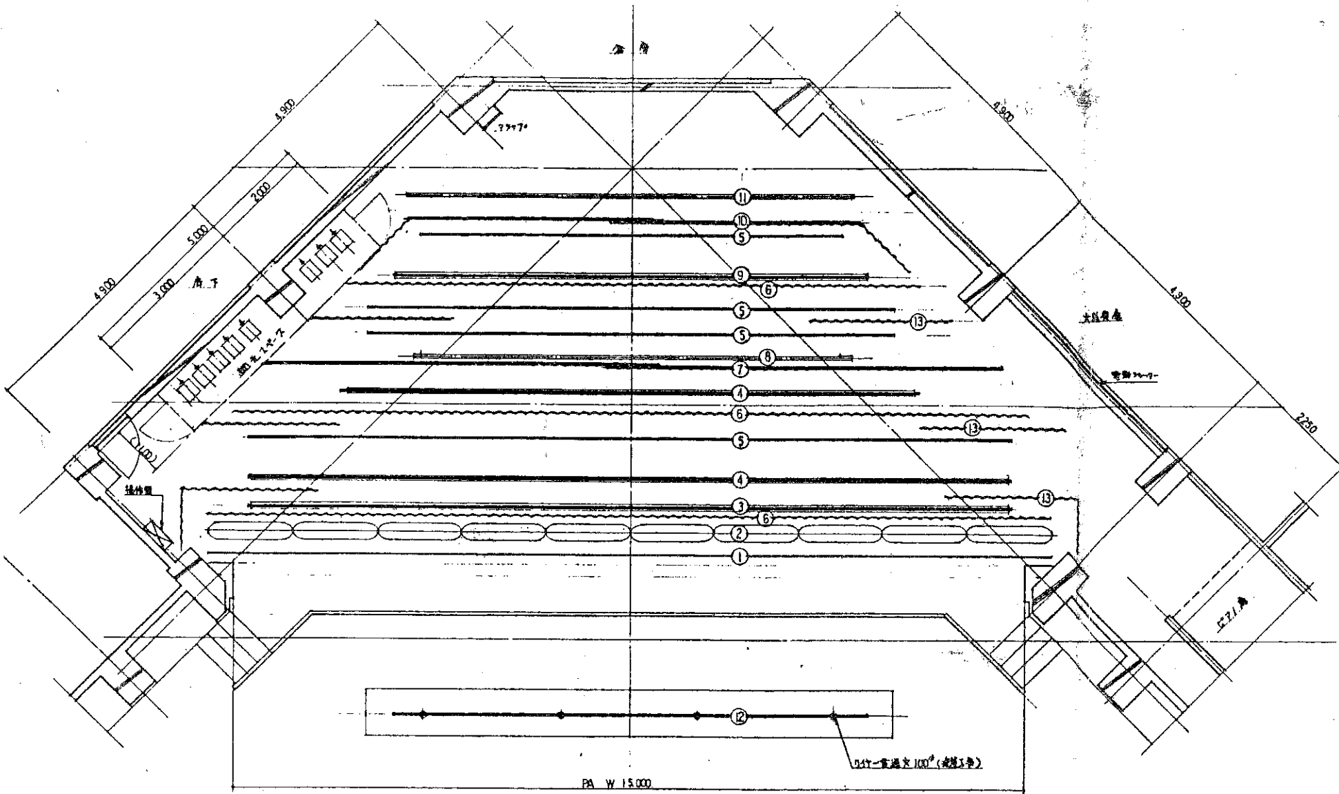
ステージ平面図 1:50
