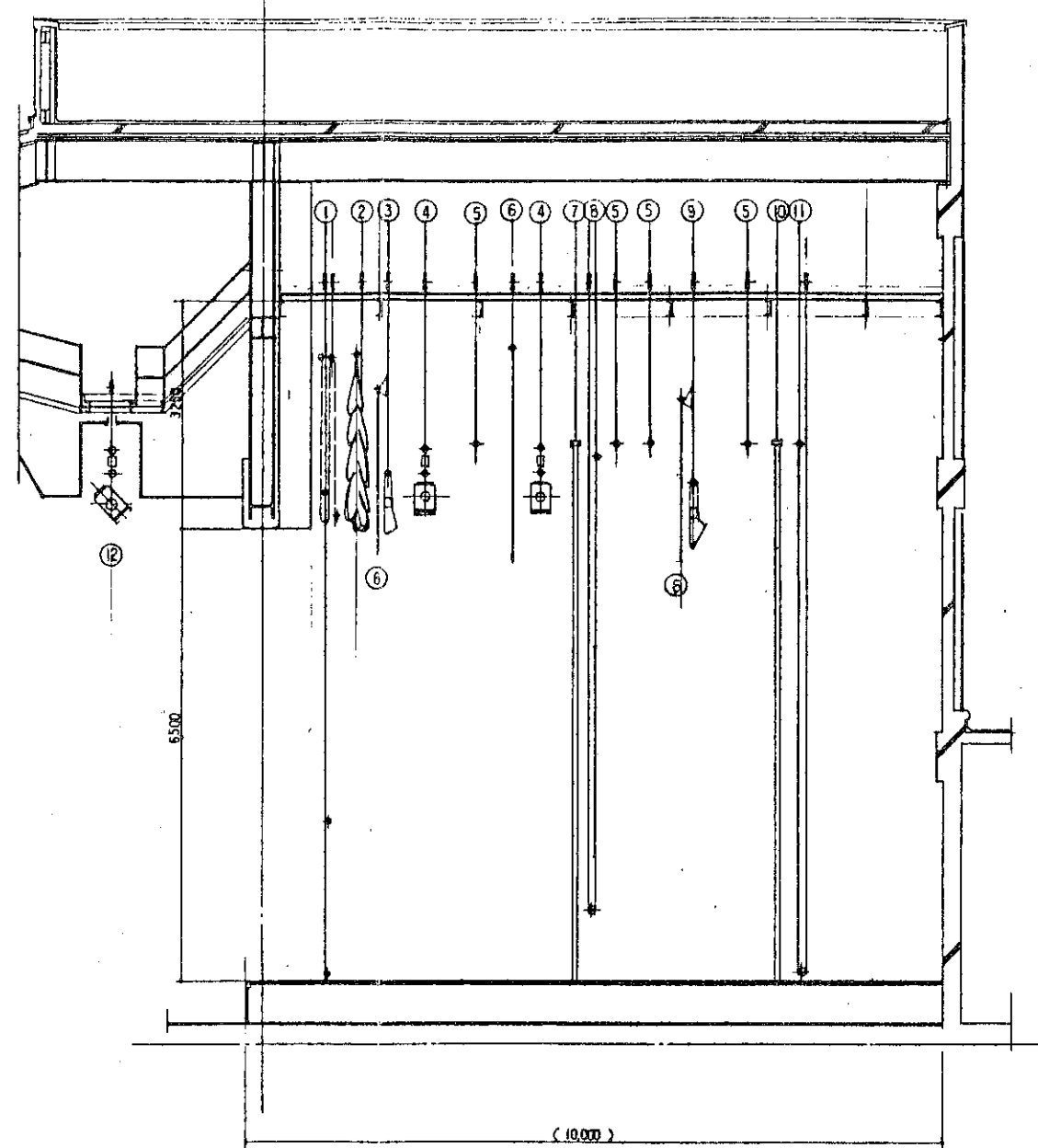
ステージ断面図 1:50
